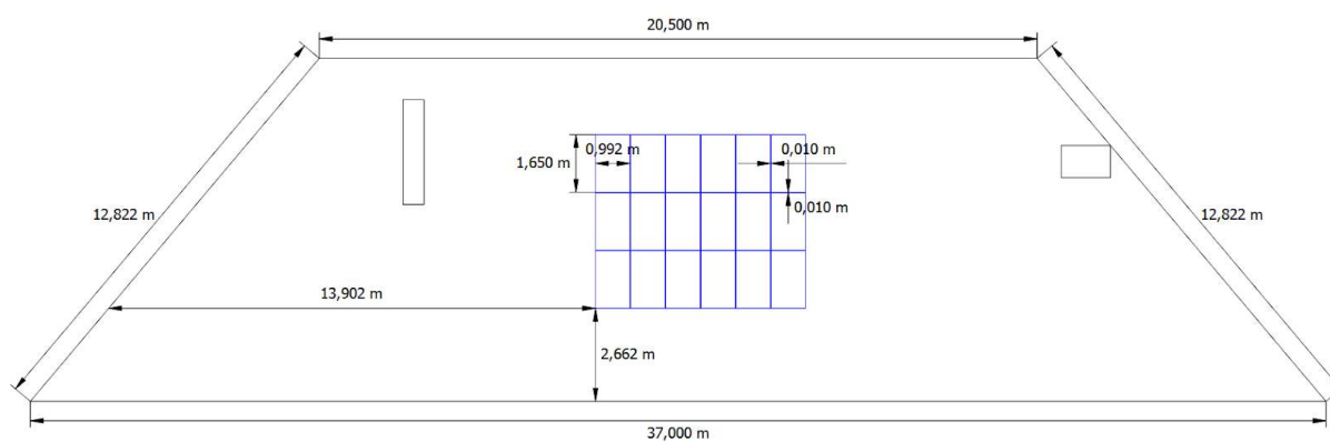
Rys. 6. Obszar posadowienia instalacji na zachodniej połaci dachu
