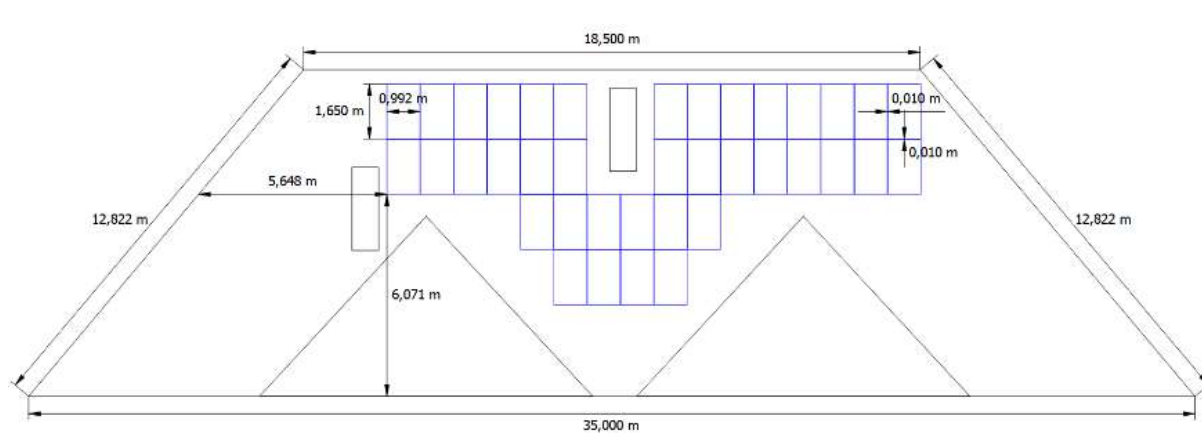
Rys. 4. Obszar posadowienia instalacji na południowej połaci dachu
