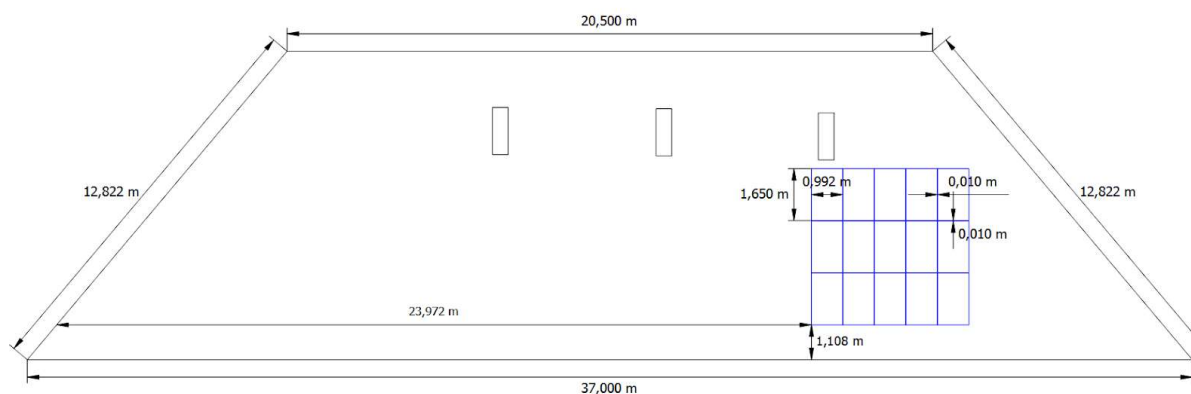
Rys. 4. Obszar posadowienia instalacji na południowej połaci dachu
