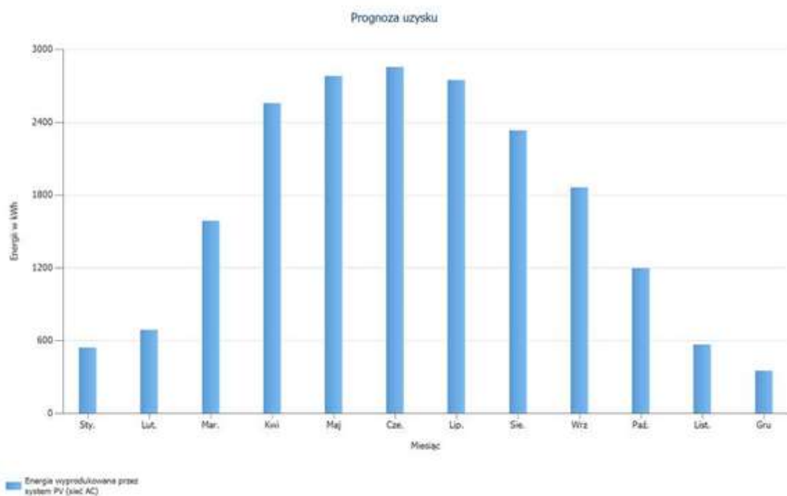
Rys. 10. Uzyski energii z instalacji fotowoltaicznej
