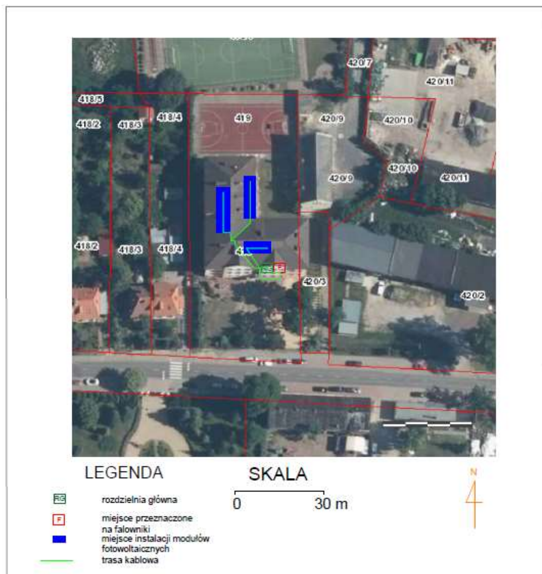
Rys. 8. Lokalizacja falownika, rozdzielni głównej oraz przebieg trasy kablowej
